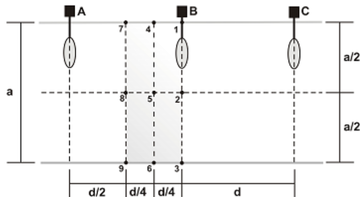
Figura C.1. Distribución unilateral
